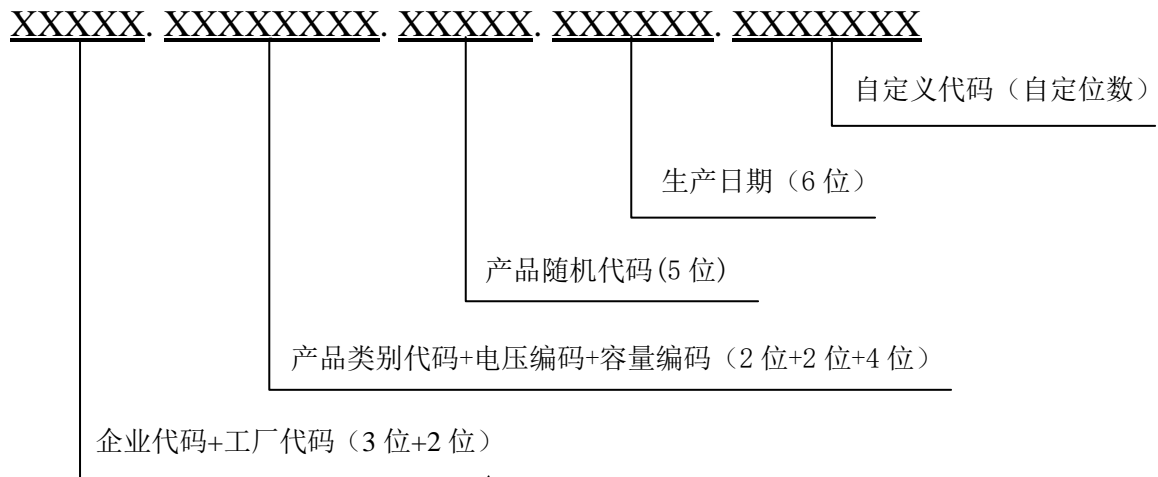
图1 二维码编码规则结构示意图
